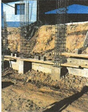
Foto 1: Finalización de cimiento de 1.00M de profundidad bajo el nivel del terreno natural. Del lado sur del centro educativo.
