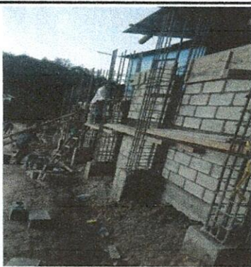
Foto 3: Fundición de columnas de concreto armado de 0.60 x 0.40 Metros.
